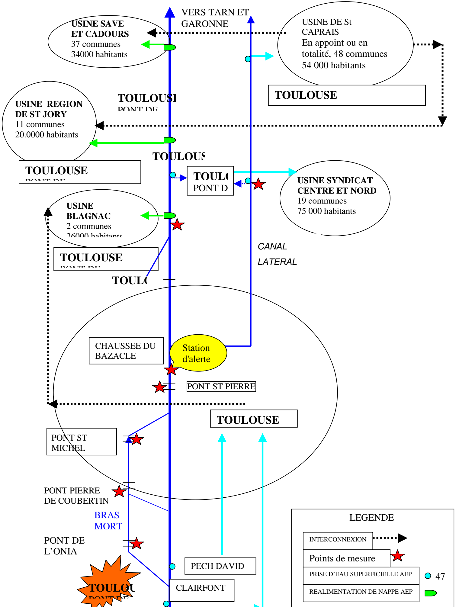
Figure 9 : Synoptique du réseau d'alimentation en eau potable dans la zone de l'accident
